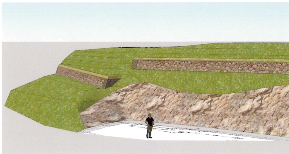
土嚢+斜面のケース
