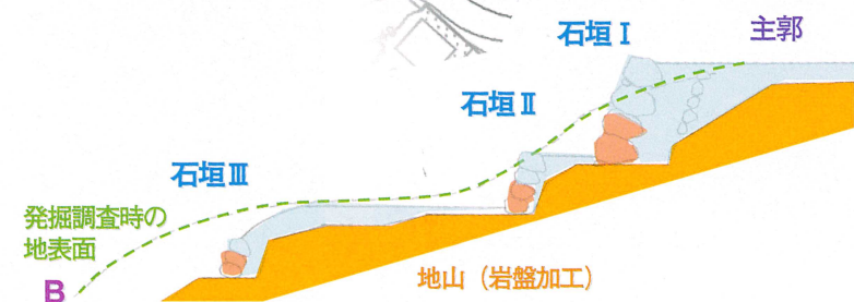
A-Bラインの石垣Ⅰ～Ⅲ断面模式図
