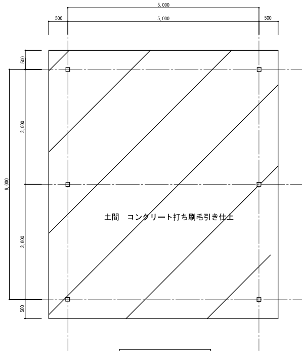
平面図 S=/50
