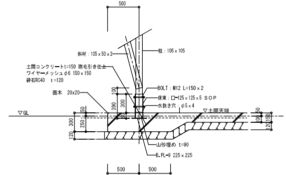
基礎詳細図 S=1/30
