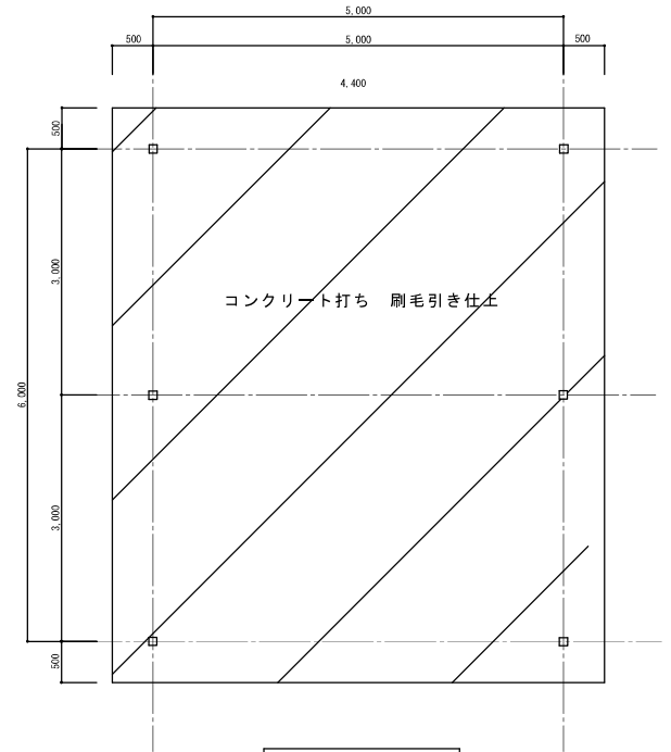
基礎伏図 S=/50
