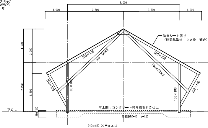
軸組図 S=/50
