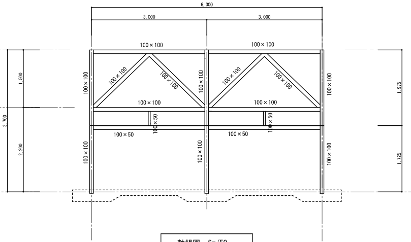
軸組図 S=/50
