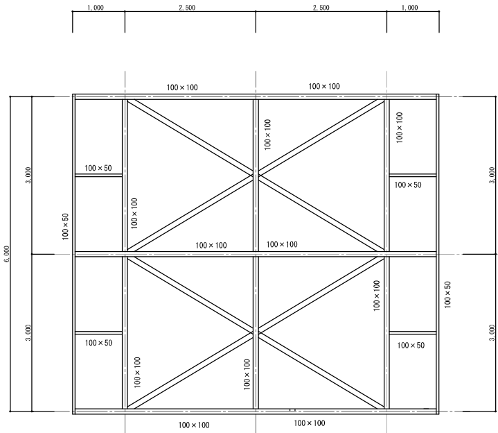
小屋伏図 S=/50
