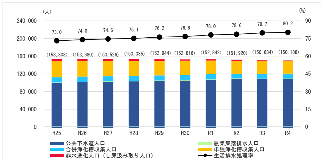
図1 生活排水処理形態別人口の推移
