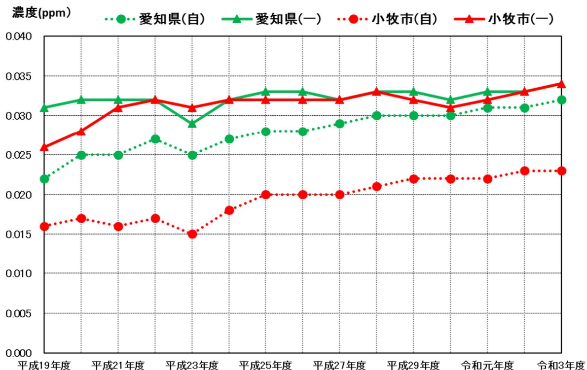
図3 光化学オキシダント 昼間年平均値
